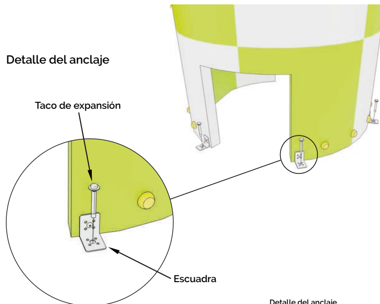
Detalle del anclaje
