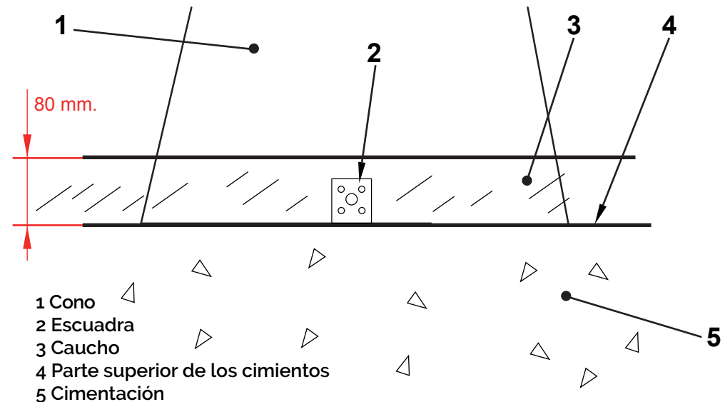
Detalle del anclaje
