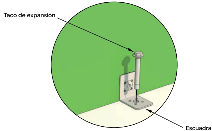
Detalle del anclaje
