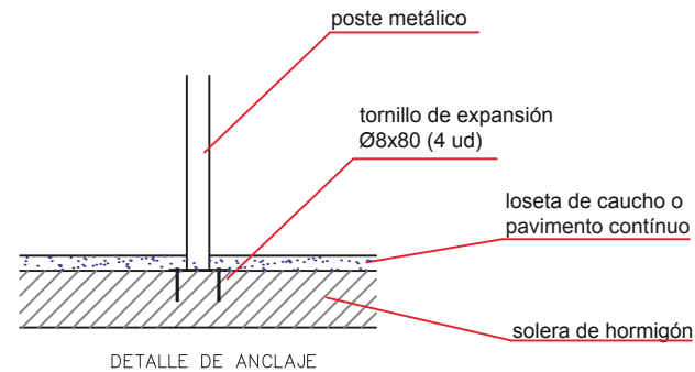
ESQUEMA DE CIMENTACIÓN EN HORMIGÓN
