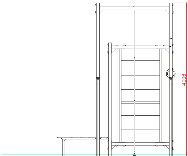
ALZADO
