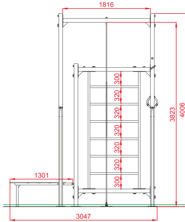
ALZADO
