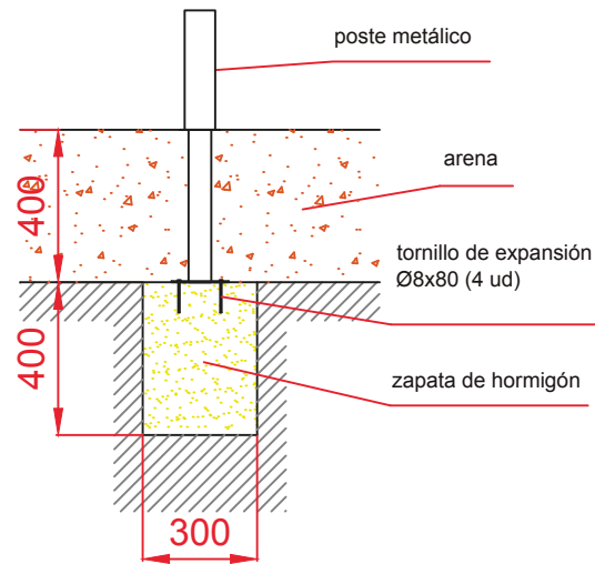
ESQUEMA DE CIMENTACIÓN EN ARENA
