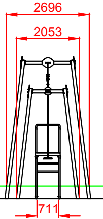
PERFIL
