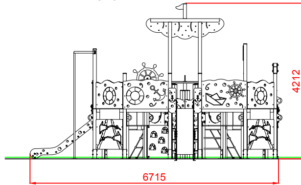
PERFIL DERECHO
