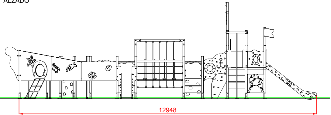
ALZADO
