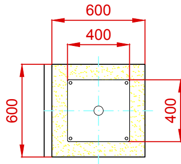
CIMENTACIÓN
