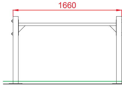
ALZADO
