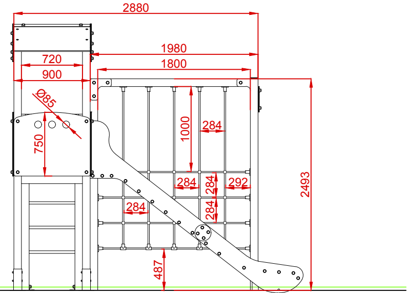
PERFIL IZQUIERDO
