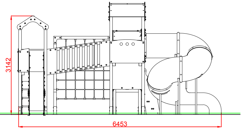
PERFIL DERECHO
