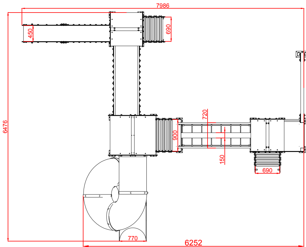
PLANTA
