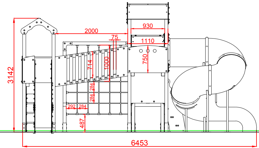
PERFIL DERECHO
