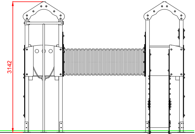
PERFIL IZQUIERDO
