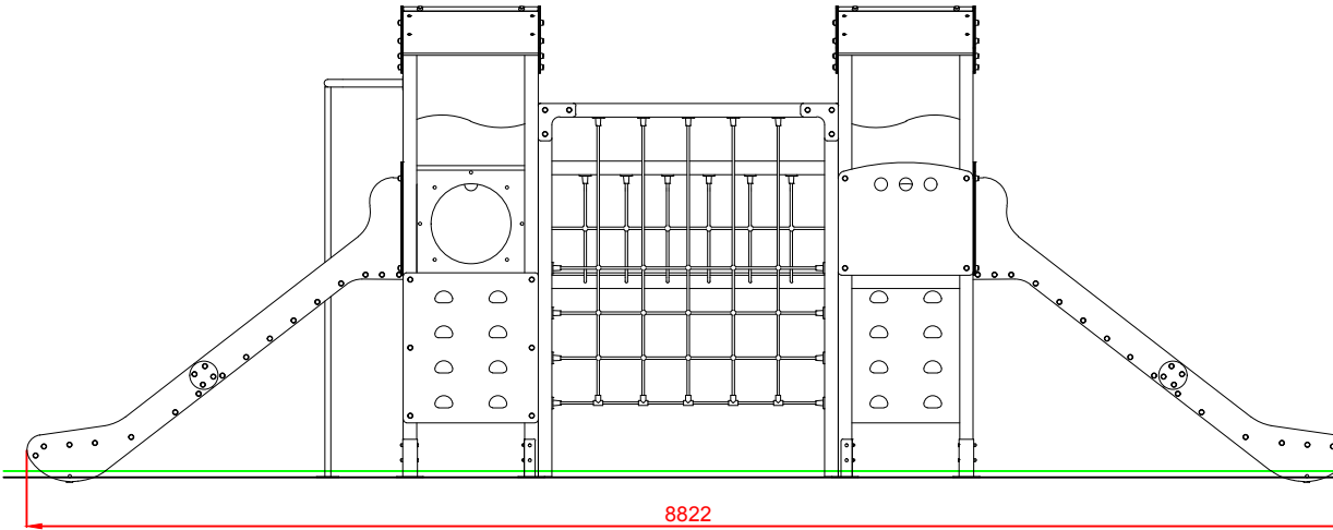
ALZADO
