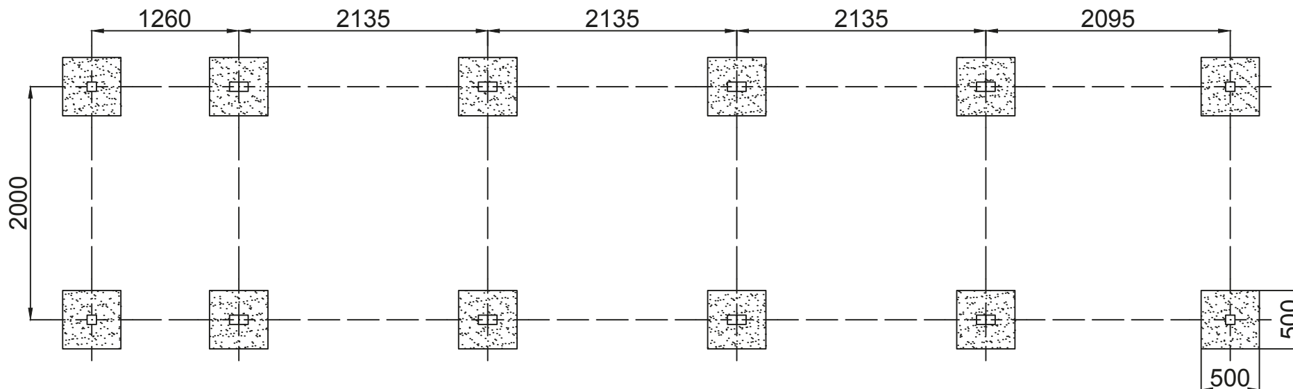
PLANTA CIMENTACIÓN
