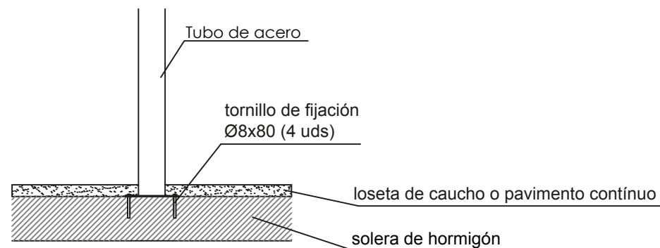
ESQUEMA DE CIMENTACIÓN PLACAS EN HORMIGÓN
