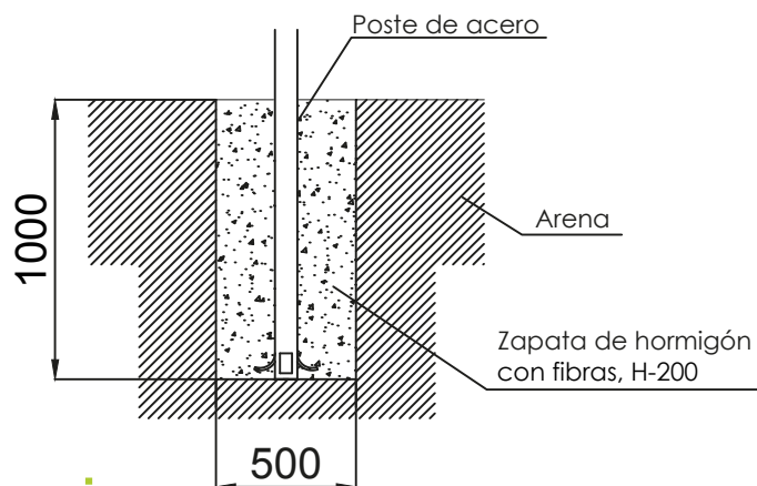
ESQUEMA DE CIMENTACIÓN POSTES
