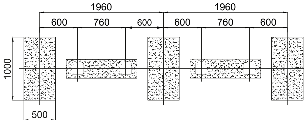
ESQUEMA DE CIMENTACIÓN PLACAS EN HORMIGÓN
