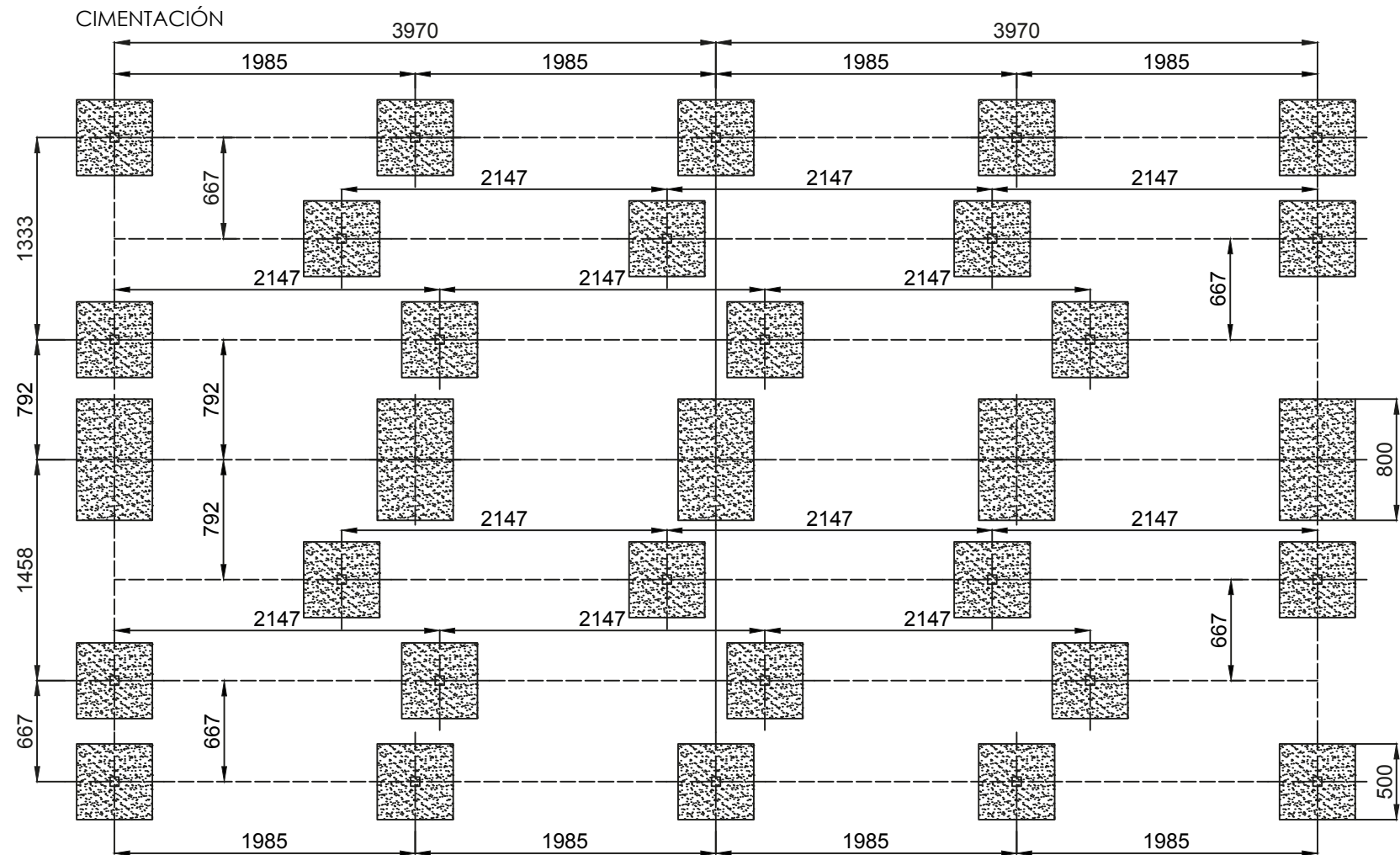
ESQUEMA DE CIMENTACIÓN EN HORMIGÓN
