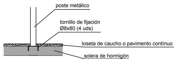
ESQUEMA DE CIMENTACIÓN EN HORMIGÓN
