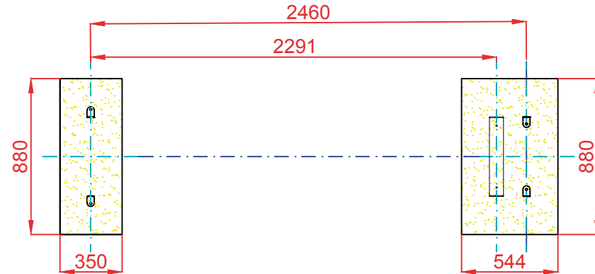
PLANTA CIMENTACIÓN
