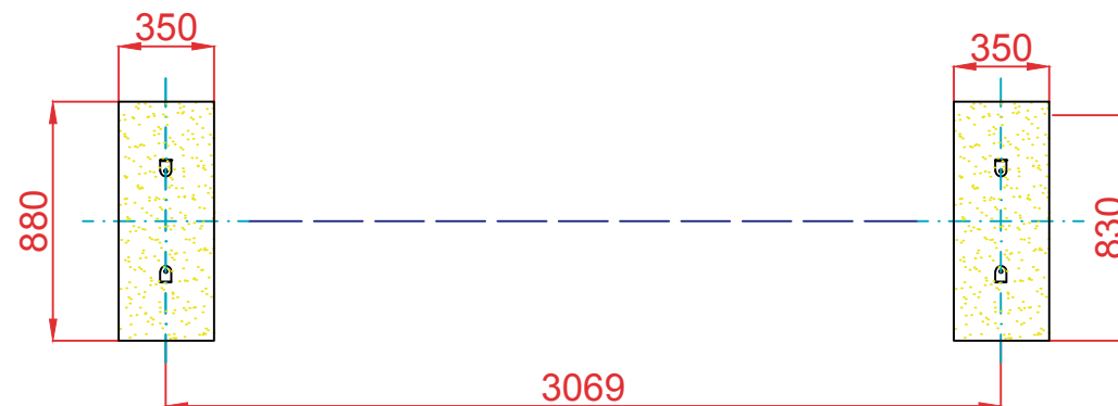
PLANTA CIMENTACIÓN
