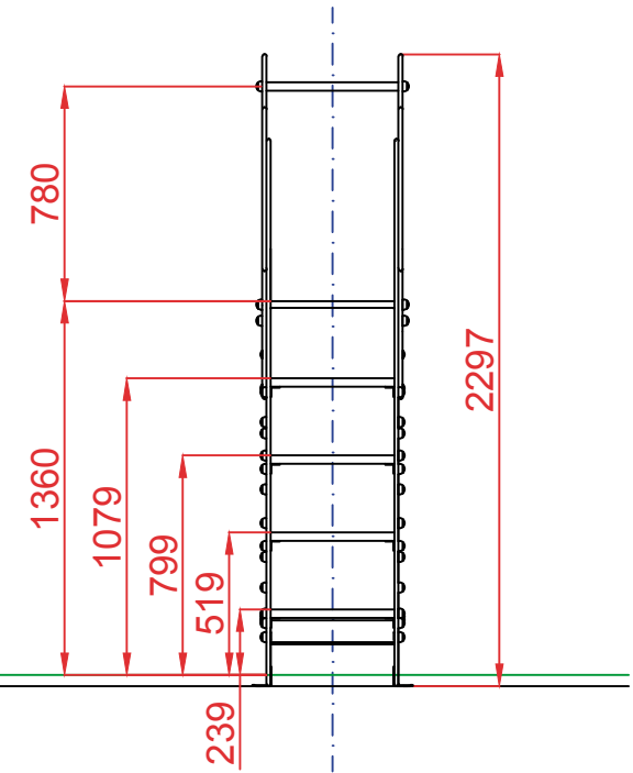
PERFIL
