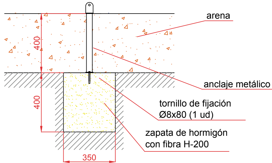
ESQUEMA DE CIMENTACIÓN EN ARENA E: 2/1
