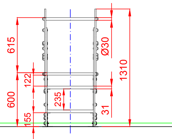
PERFIL IZQUIERDO
