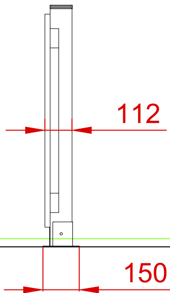
PERFIL DERECHO
