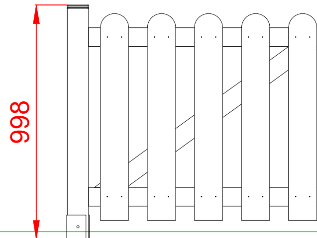
ALZADO
